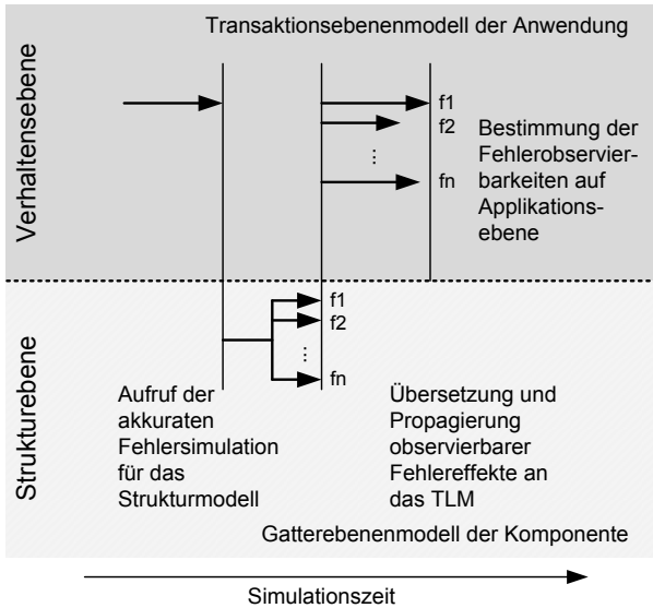
Abbildung 1. Konzeptuelle Übersicht der vorgeschlagenen ebenenübergreifenden Fehlersimulation
